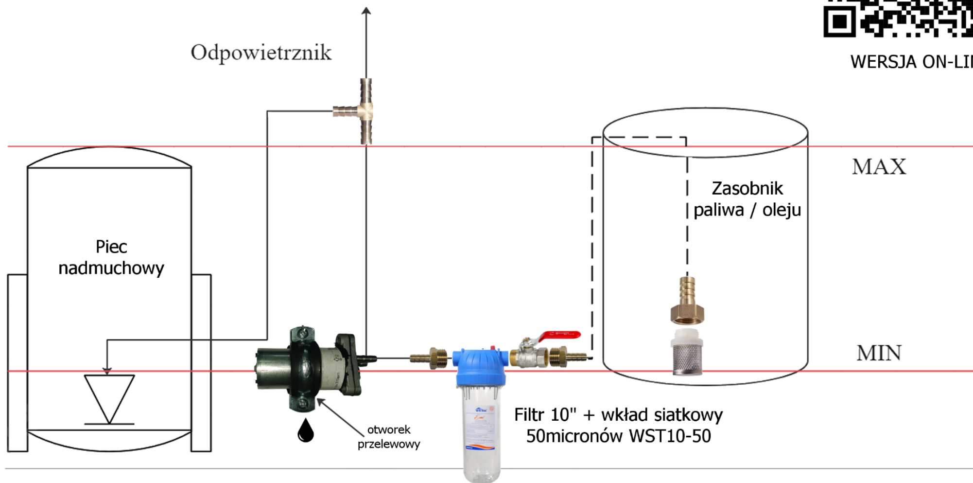
ZAWÓR HYDRAULICZNY POMPKI MPG5 W WERSJI Z BECZKĄ
