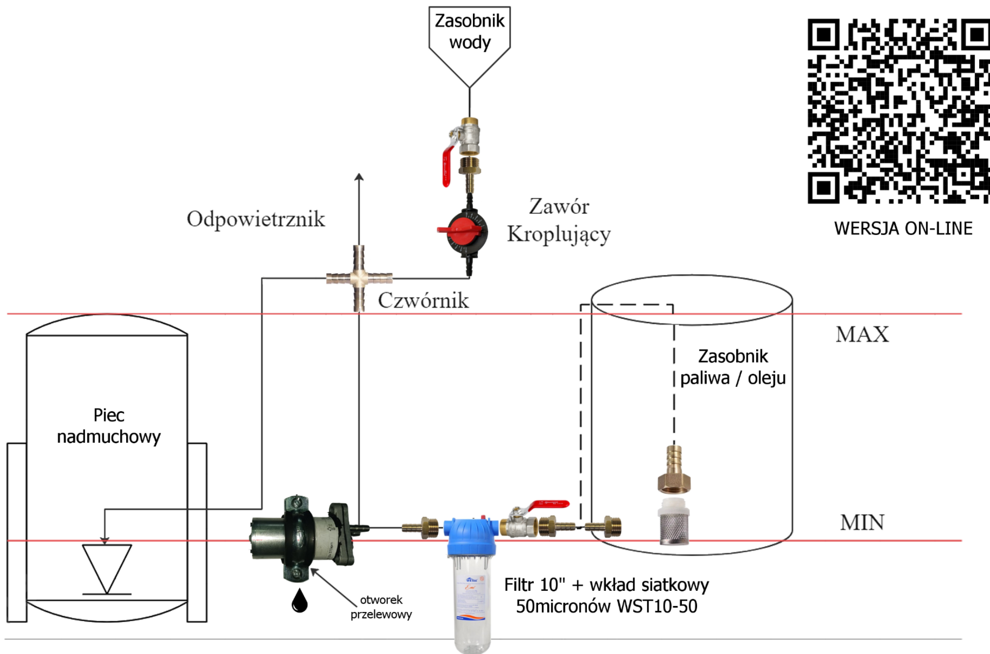
SYSTEM AUTOMATYCZNEGO OCZYSZCZANIA SADZY ZAWÓR HYDRAULICZNY POMPKI MPG5 W WERSJI MAUSER LUB BECZKA
